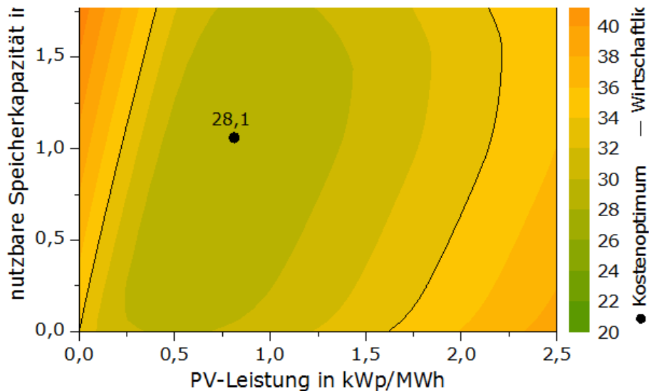
Abbildung 3: Mittelfristiges und langfristiges Szenario, wieder in Form der mittleren Stromkosten (siehe Abbildung 2). Im mittelfristigen Szenario sinken die PV-Systemkosten auf 1.200 €/kWp, die Batteriespeicherkosten auf 1.000 €/kWh, die Einspeisevergütung auf 6 ct/kWh. Im langfristigen Szenario sinken sie auf 1.000 €/kWp, 600 €/kWh, 2 ct/kWh.
