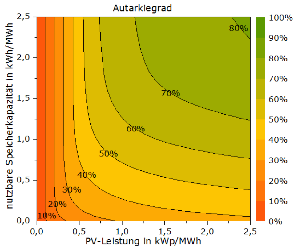
Abbildung 1: Eigenverbrauchsanteil und Autarkiegrad in Abhängigkeit der nutzbaren Speicherkapazität und PV-Leistung, jeweils normiert auf den Jahresstrombedarf in MWh. Durch die Normierung lassen sich die Bewertungsgrößen für Haushalte je nach der Höhe des Jahresstrombedarfs abschätzen.
