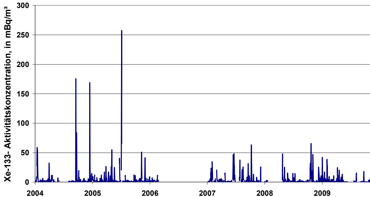
Abbildung 1.1-1 Zeitreihe der Xe-133-Aktivitätskonzentration in den Jahren 2004 bis 2009 an der IMS-Station RN33 auf dem Schauinsland (Time series of Xe-133-activity concentration at IMS-station RN33 at Schauinsland mountain for the years 2004 to 2009)
