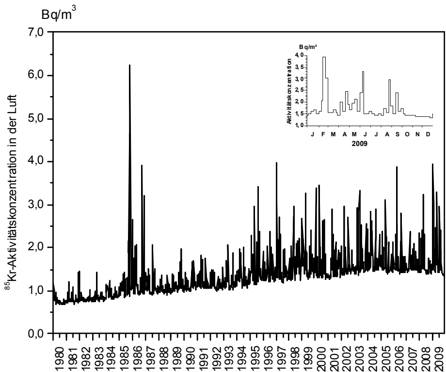
Abbildung 2.1.1-2 Aktivitätskonzentrationen von Kr-85 in der bodennahen Luft am Probenentnahmeort Freiburg (Activity concentrations of Kr-85 in air close to ground level at the sampling location Freiburg)
