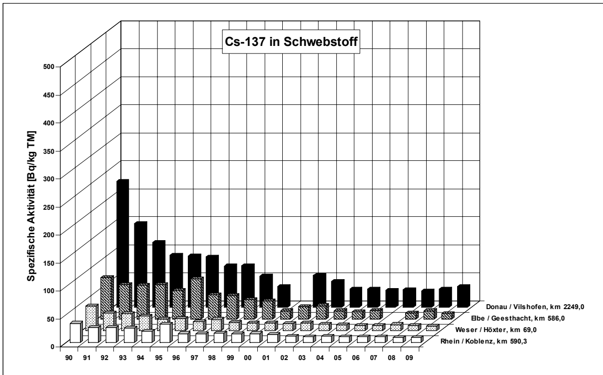
Abbildung 2.2.2-6 Spezifische Aktivitäten (Bq/kg TM) von Cs-137 in Schwebstoffproben ausgewählter Binnengewässer (Jahresmittelwerte) (Cs-137 specific activities for samples of suspended matter in Bq/kg TM from selected inland waters - annual mean values)
