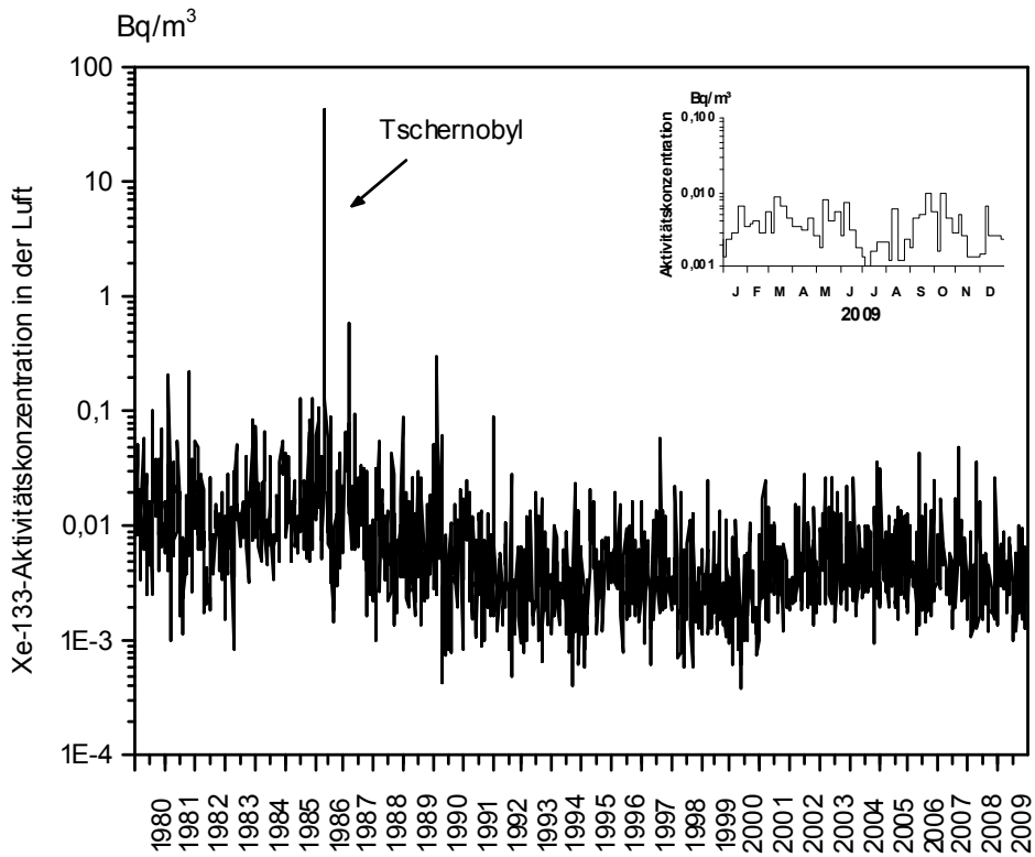
Abbildung 2.1.1-1 133 Xe-Aktivitätskonzentration in der bodennahen Luft am Probenentnahmeort Freiburg ( 133 Xe-activity concentration in air close to ground level at the sampling location Freiburg)
