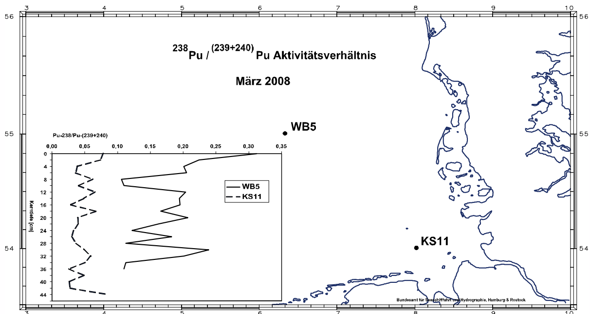
Abbildung 2.2.1-16 Profil des Verhältnisses der Pu-238- und Pu-(239+240)-Aktivitäten in Sedimentkernen aus der Deutschen Bight im März 2008 (Profiles of activity ratios of Pu-238- and Pu(239+240) in sediment cores from the German Bight in March 2008)
