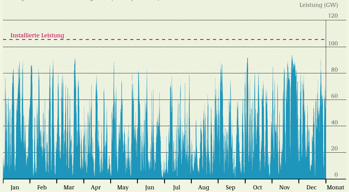
Einspeisezeitreihe von Wind gesamt (Meteo-Jahr 2009)
