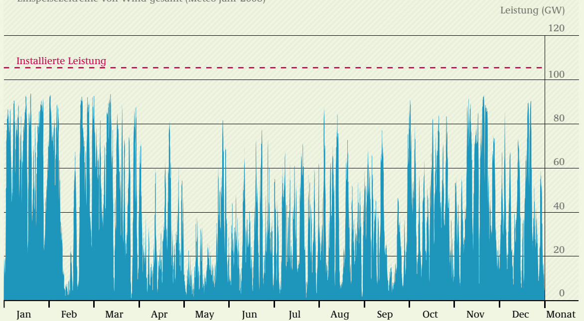
Einspeisezeitreihe von Wind gesamt (Meteo-Jahr 2008)
