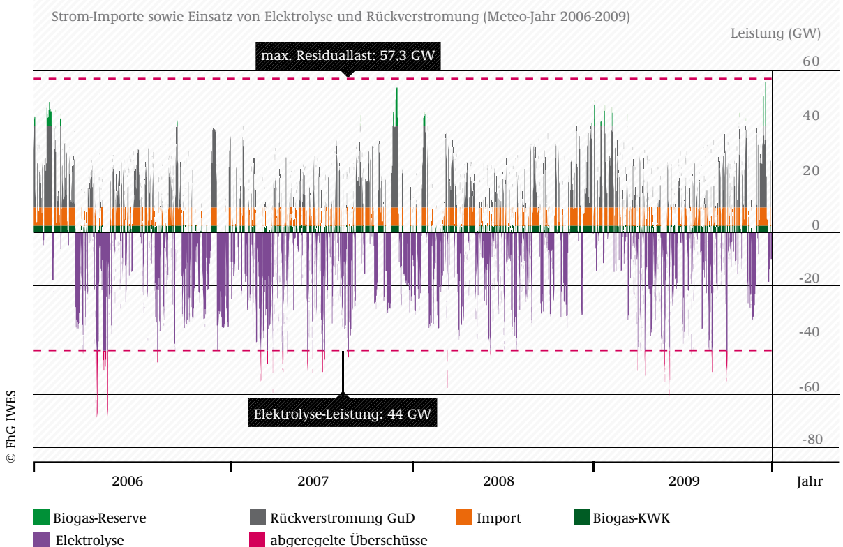
ABB 7-27 VERLAUF DER RESIDUALEN GESAMTLAST UND EINSATZ VON SPEICHERN UND RESERVEKRAFTWERKEN FÜR DEN BETRACHTUNGSZEITRAUM MIT DEN METEO-JAHREN 2006-2009
