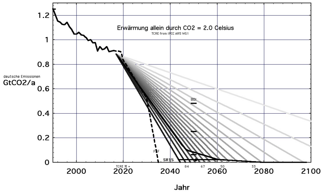
Abb. 8.1. Wie Abbildung 7a1 , aber für das 2-Grad-Ziel. Das Klimaschutzgesetz und der stärkste BDI-Reduktionspfad erreichen das 2.0-Grad-Ziel mit weniger als 67% Wahrscheinlichkeit.
