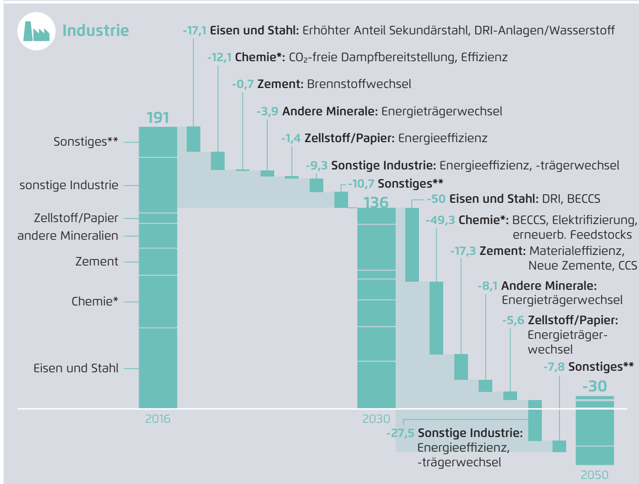
Treibhausgasminderungen in der Industrie nach Branchen im Szenario KNmin zwischen 2016 und 2030 sowie zwischen 2030 und 2050 (Mio. t CO 2 -Äq.)
