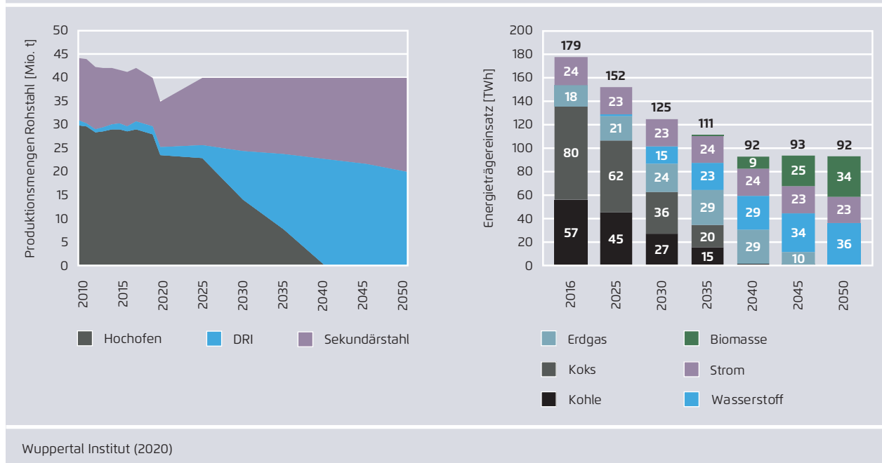
Rohstahlproduktion nach Routen und Energieträgereinsatz 5 in der Eisen- und Stahlindustrie Abbildung 30
