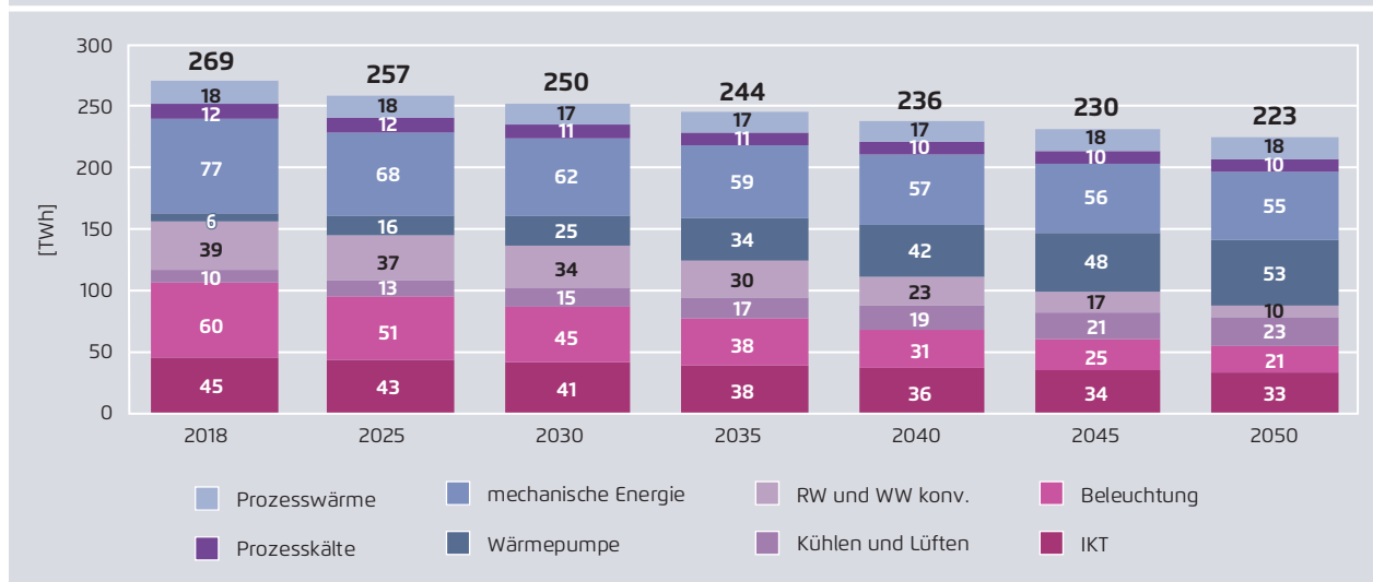
Gebäudesektor: Stromverbrauch nach Verwendungszwecken im Szenario KNmin
