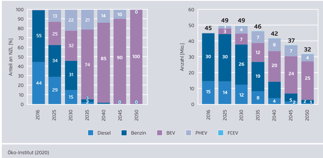
Neuzulassungen und Bestand Pkw im Szenario KNmin
