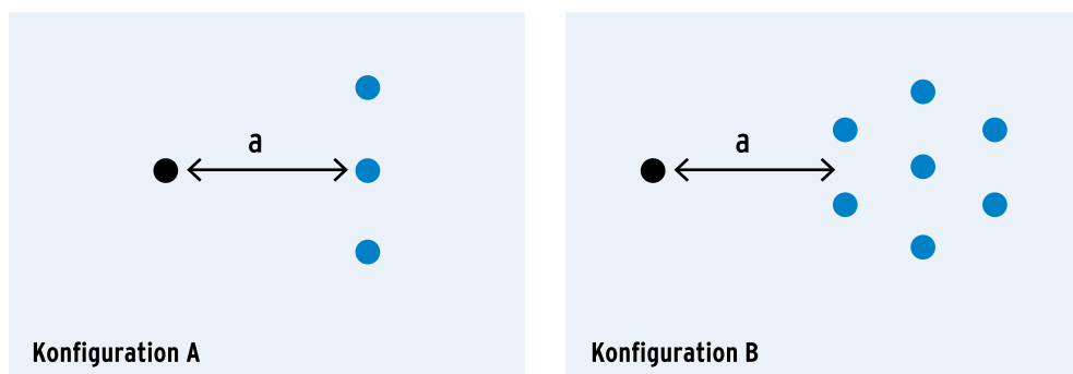
Abbildung 3: Anlagenkonfigurationen von Windparks
