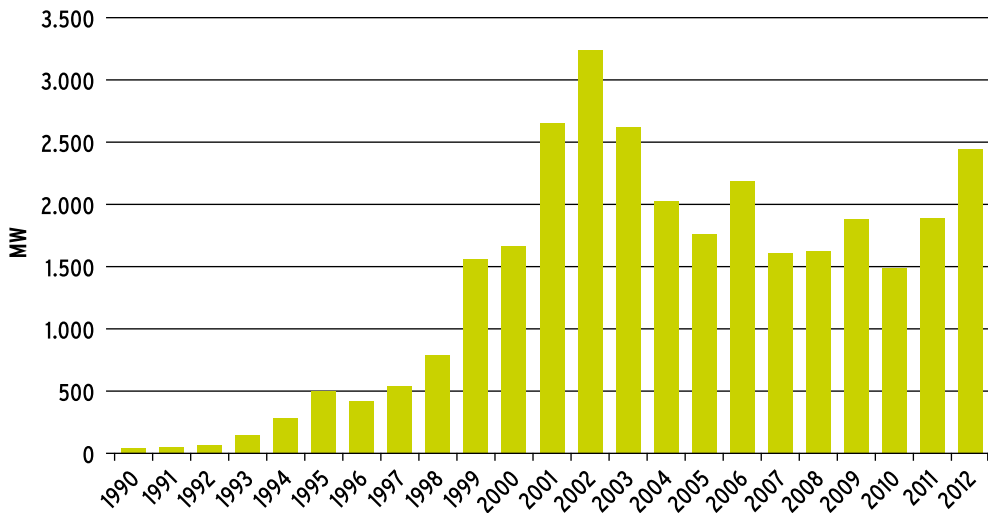
Abbildung 1: Entwicklung der jährlich neu installierten Windenergieleistung (Rückbau aufgrund von Repowering nicht berücksichtigt)
